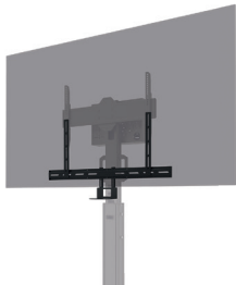
AV50-500BL Kit de support pour caméra PTZ/UC Taille de l'écran: 43-110" Capacité: 5 kg VESA: 200x200 - 800x600 Montage haut et bas
